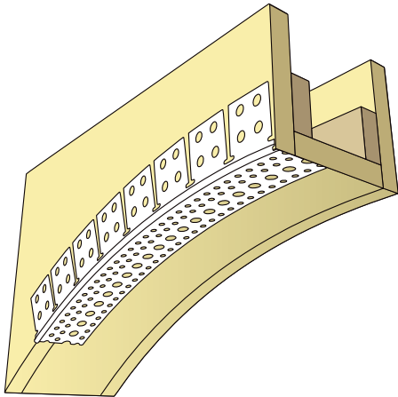
■ PEA90 DETAIL
