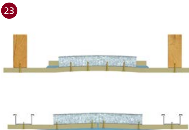
■ STITCHING BATTENS
