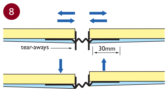
■ PEXPH30 DETAIL
