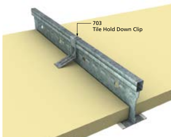
■ TILE HOLDDOWN CLIP
