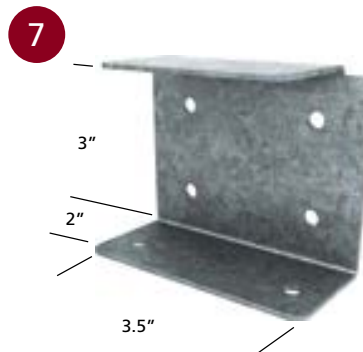
■ 202 SILL/HEADER BRACKET
